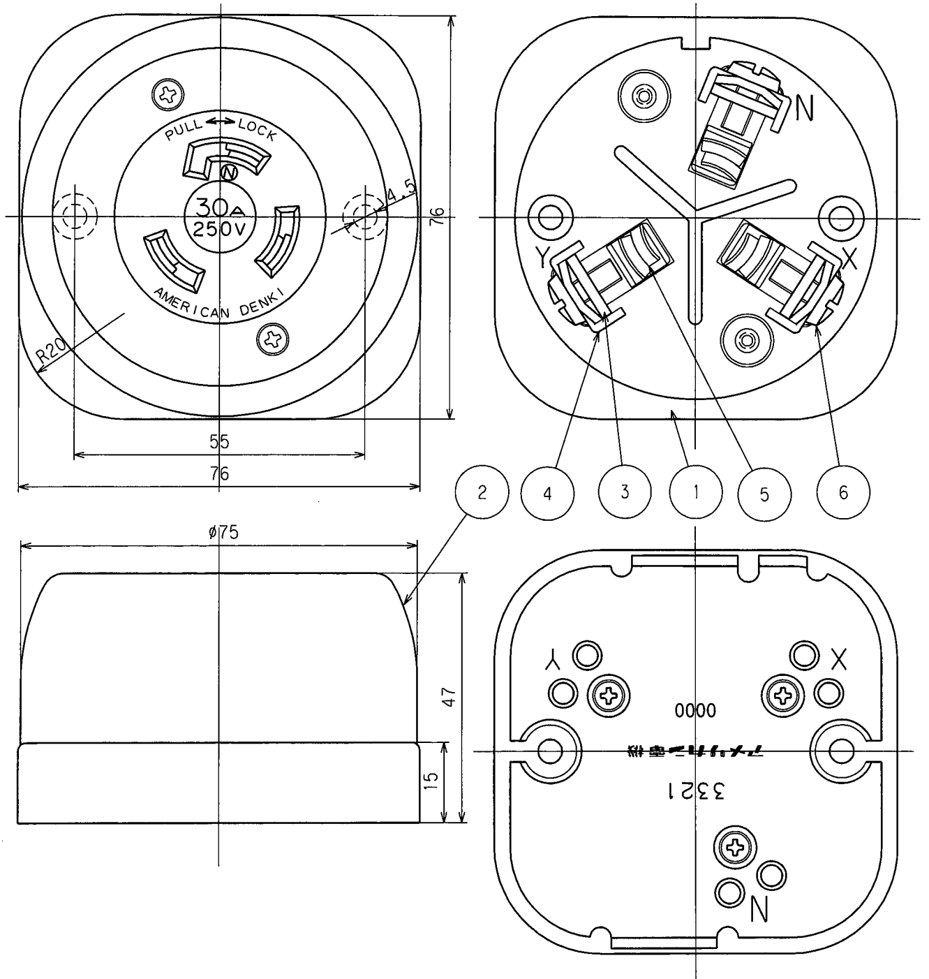
端子記号記載図
