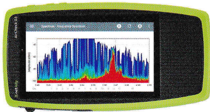
AirCheck G3のSpectrumアプリ
