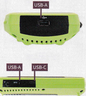
2.4/5GHz 帯用ポータブル スペクトラムアナライザ NXT-1000(オプション)
