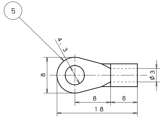
付属圧着端子詳細図(2:1)
