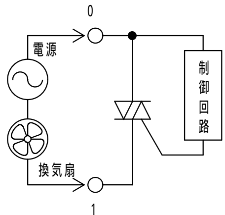
内部回路図
