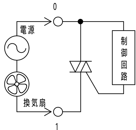
内部回路図
