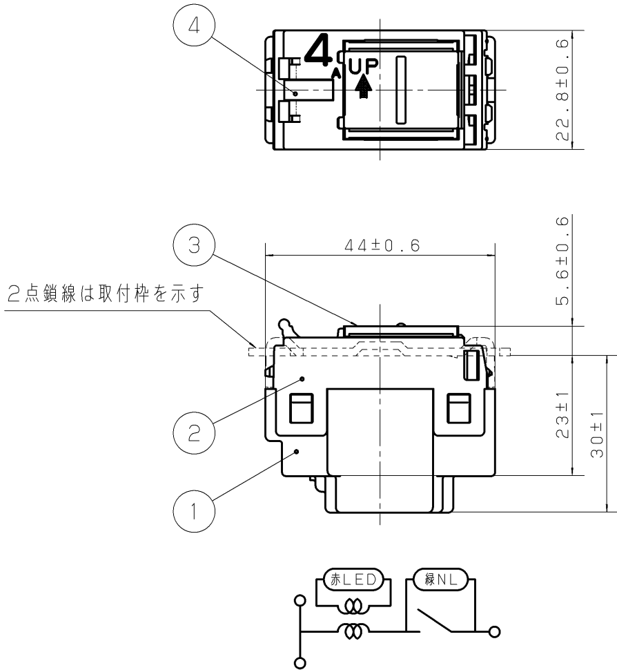
内部回路図
