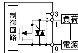
内部回路図
